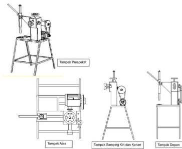
Tampak Perspektif
