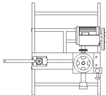
Tampak Atas
