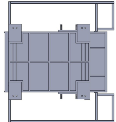
Tampak Bawah
