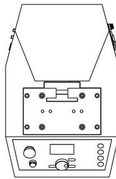
Tampak Atas
