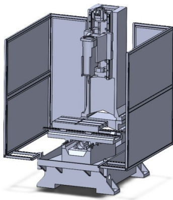
Tampak Perspektif
