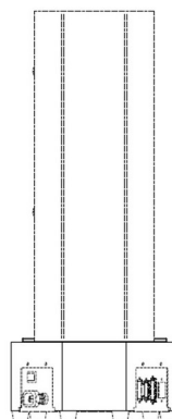
Tampak Belakang
