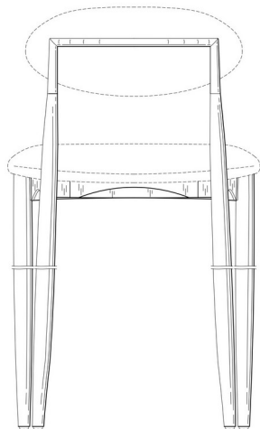
Tampak Belakang
