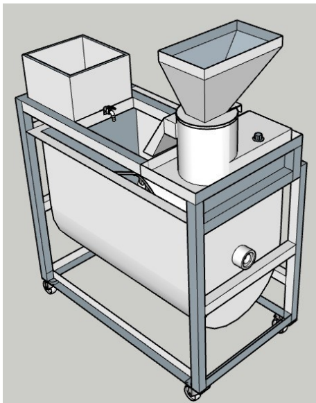
Tampak Perspektif
