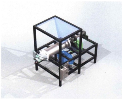
Tampak Perspektif
