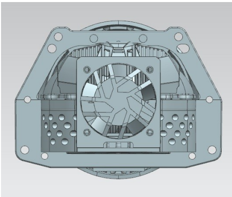
Tampak Belakang
