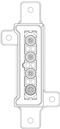
Tampak Depan
