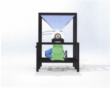
Tampak Belakang
