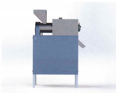
Tampak Belakang
