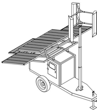
Tampak Perspektif
