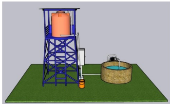
Tampak Depan
