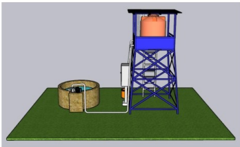
Tampak Belakang
