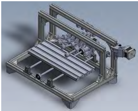
Tampak Perspektif
