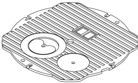
Tampak Perspektif
