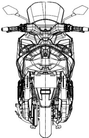
Tampak Belakang
