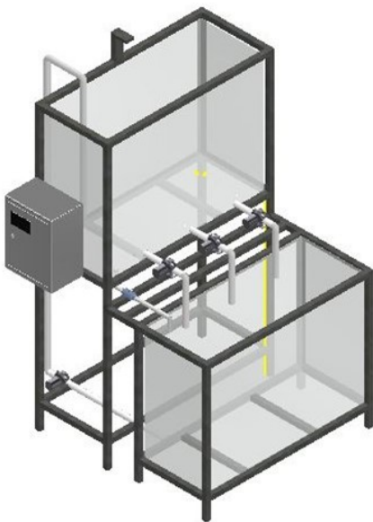
Tampak Perspektif
