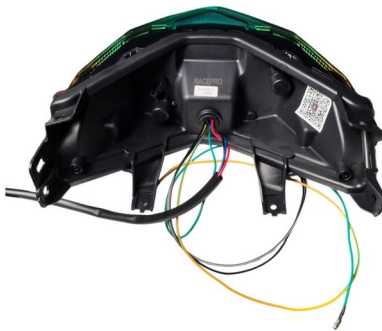
Tampak Belakang
