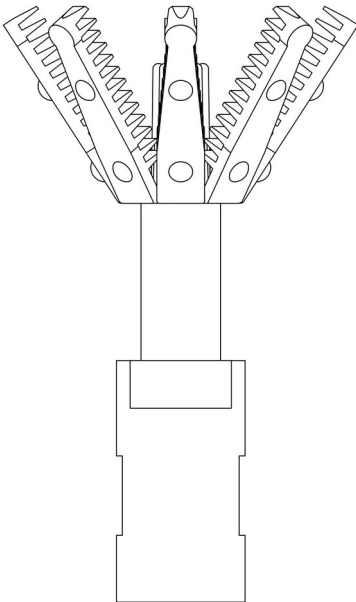
Tampak Belakang
