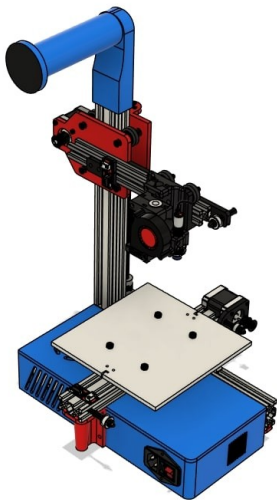
Tampak Perspektif
