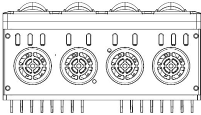
Tampak Bawah
