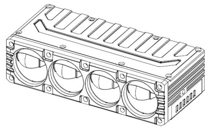
Tampak Perspektif
