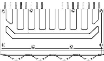
Tampak Atas
