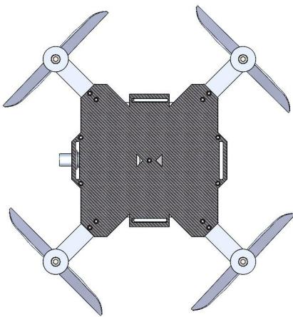
Tampak Atas
