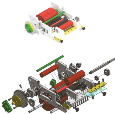
Gambar 6 : Perspektif
