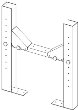
Tampak Perspektif
