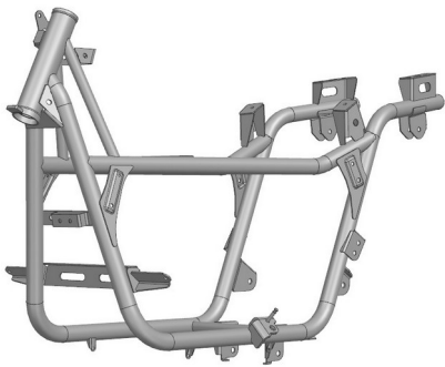
Tampak Perspektif
