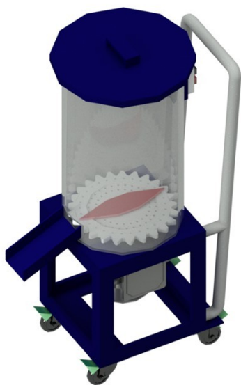
Tampak Perspektif
