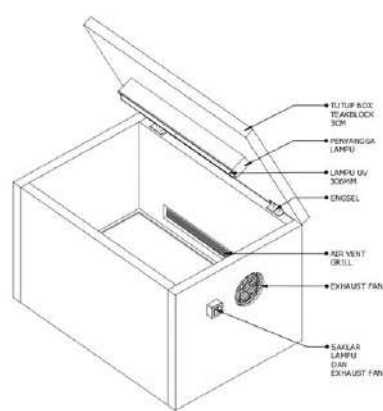
Tampak Perspektif
