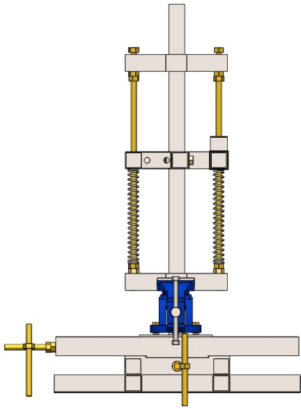
Tampak Depan
