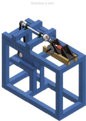
Gambar 6 : Perspektif
