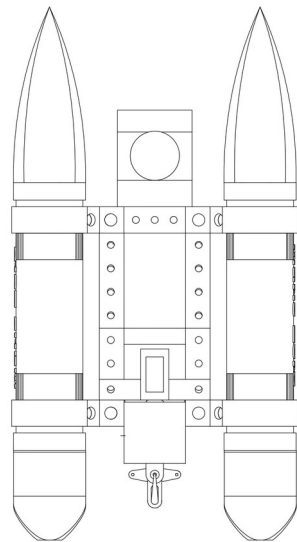
Tampak Bawah
