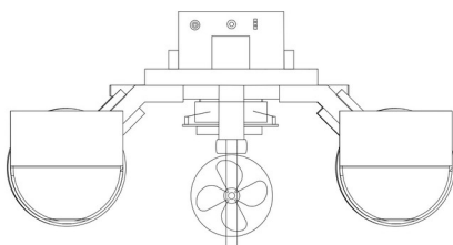
Tampak Belakang
