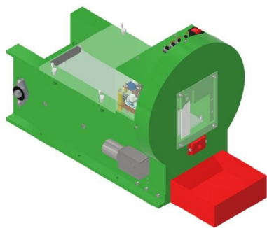
Tampak Perspektif
