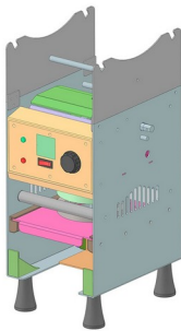
Tampak Perspektif
