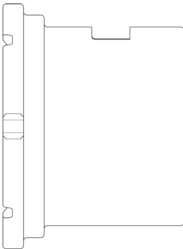
Tampak Belakang
