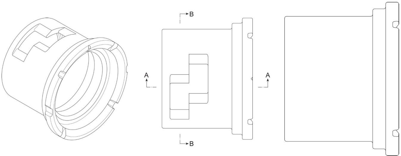
Tampak Perspektif
