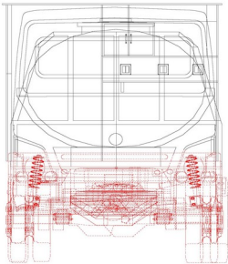
Tampak Depan
