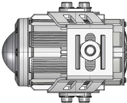
Tampak Bawah
