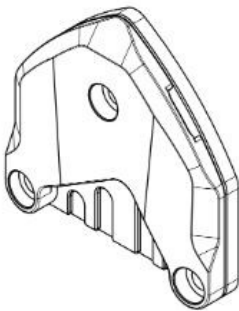
Tampak Perspektif
