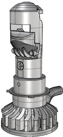
Tampak Perspektif
