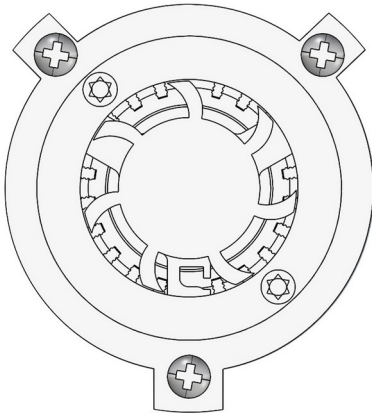
Tampak Atas
