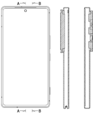
Tampak Depan
