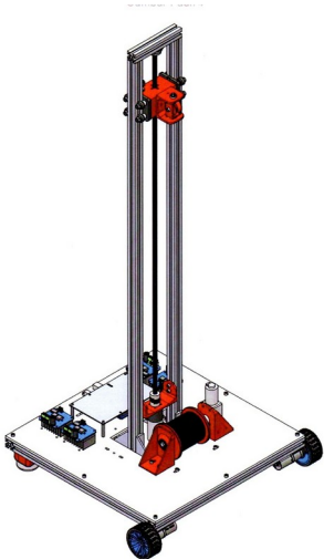
Tampak Perspektif
