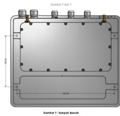
Tampak Bawah
