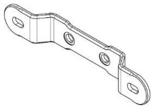
Tampak Perspektif
