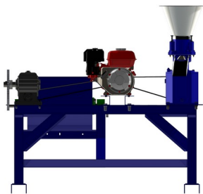
Tampak Depan
