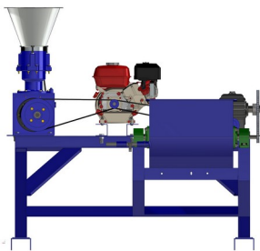
Tampak Belakang
