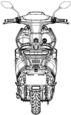
Tampak Belakang
