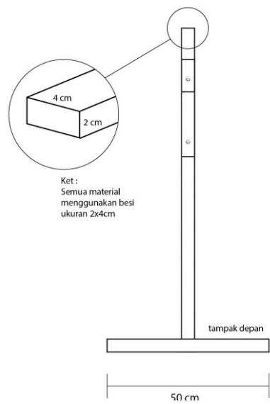
Tampak Depan
