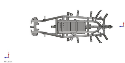
Tampak Bawah
