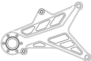
Tampak Depan
