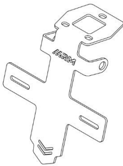
Tampak Perspektif
