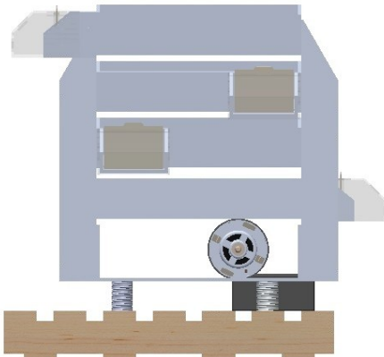
Tampak Belakang
