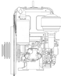
Tampak Belakang
