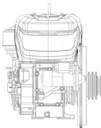
Tampak Depan
