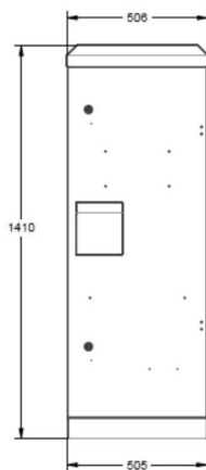
Tampak Belakang
