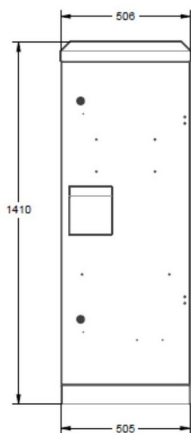
Tampak Depan
