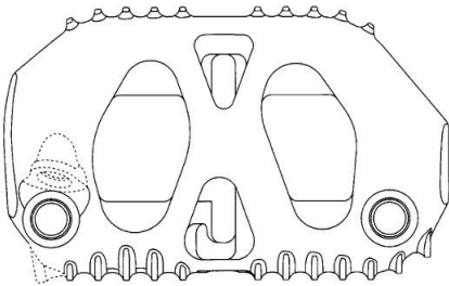
Tampak Atas
