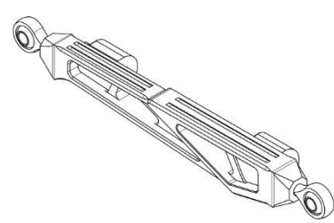
Tampak Perspektif
