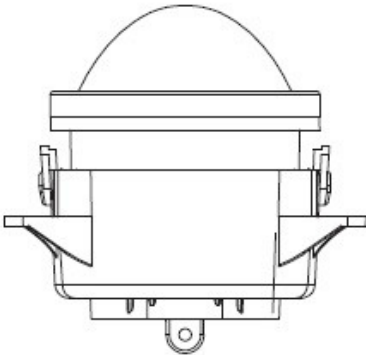
Tampak Atas
