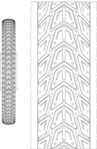
Tampak Depan
