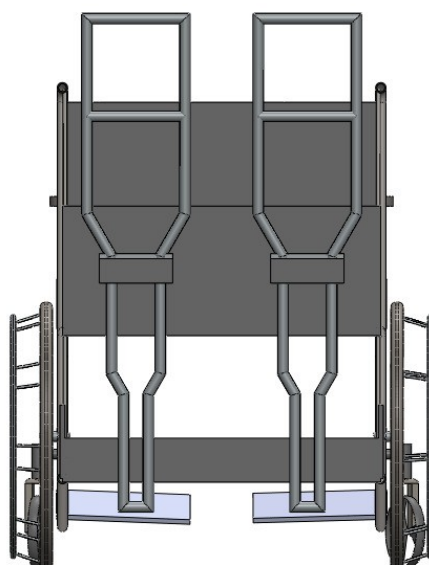
Tampak Atas
