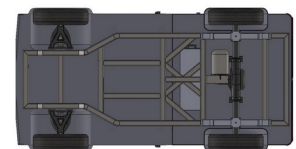
Tampak Bawah
