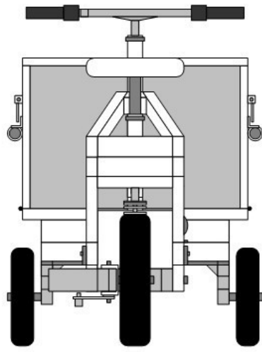
Tampak Belakang
