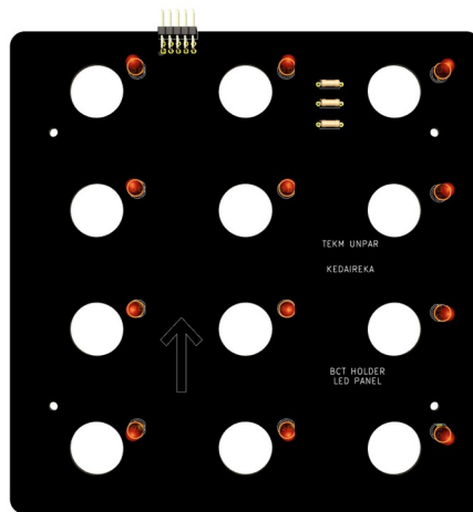
Tampak Atas
