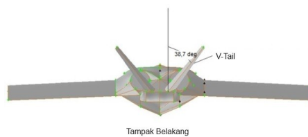
Tampak Belakang
