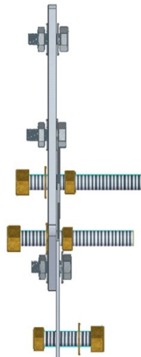
Gambar 3 : Tampak Bawah
