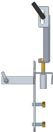
Gambar 2 : Tampak Atas
