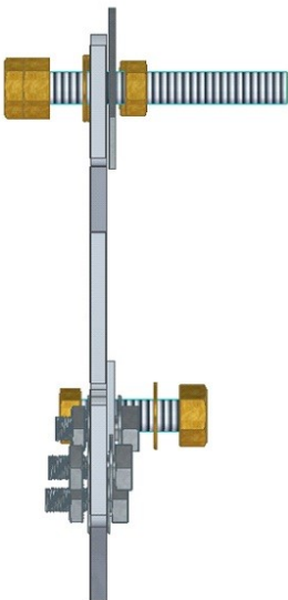
Gambar 4 : Tampak Depan
