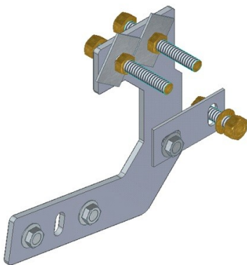
Gambar 1 : Tampak Perspektif
