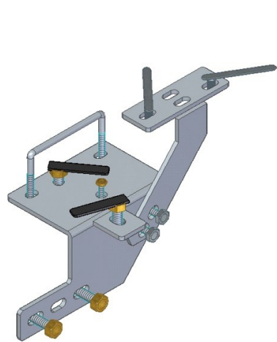
Gambar 1 : Tampak Perspektif
