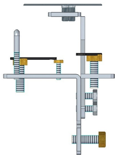
Gambar 4 : Tampak Depan
