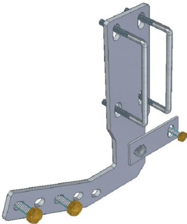
Gambar 1 : Tampak Perspektif
