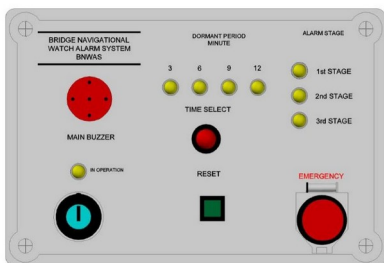
Tampak Depan
