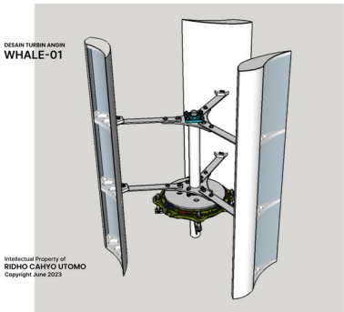
Tampak Perspektif
