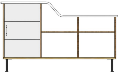
Tampak Belakang
