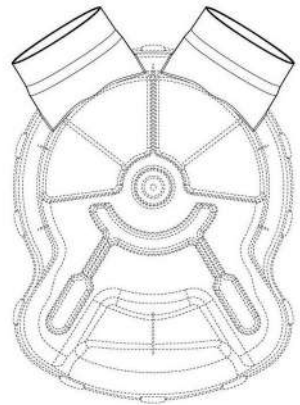
Tampak Bawah
