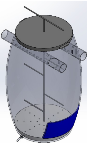
Tampak Perspektif
