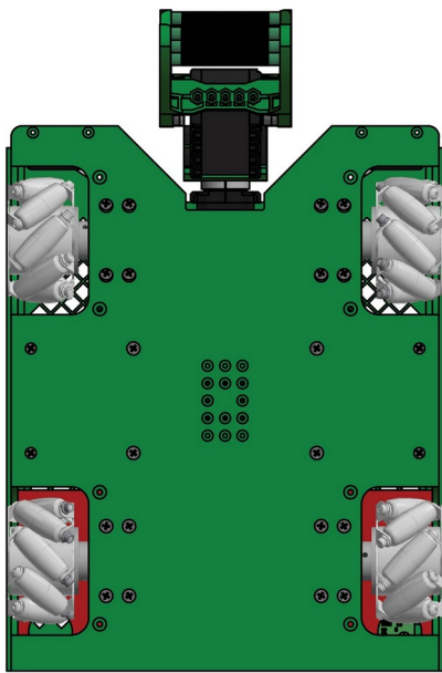
Tampak Bawah
