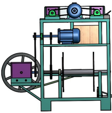
Tampak Belakang
