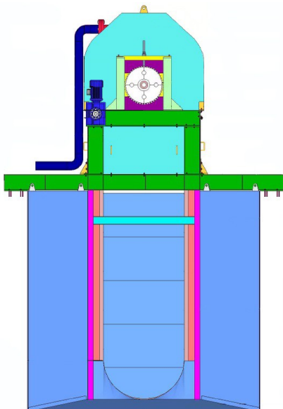
Tampak Depan
