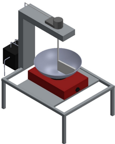
Tampak Perspektif
