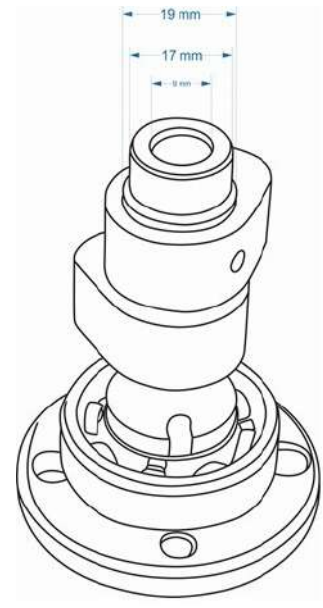
Tampak Bawah
