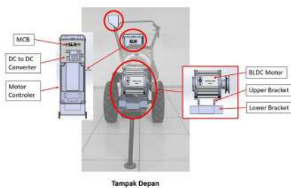
Tampak Depan
