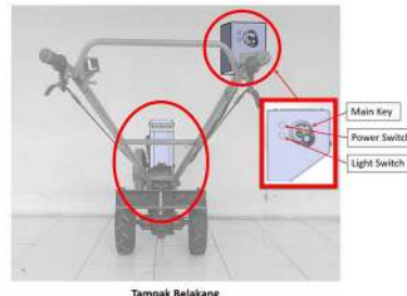
Tampak Belakang
