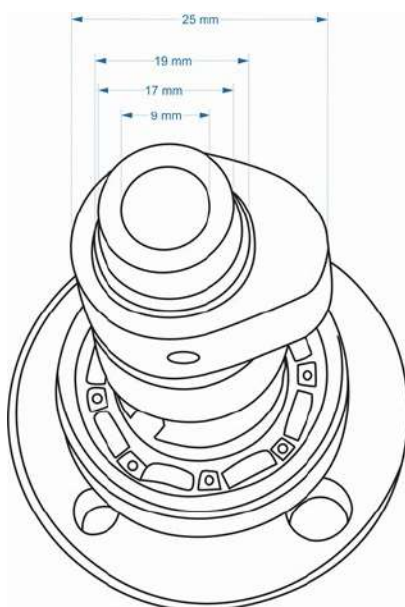
Tampak Depan
