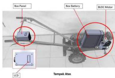
Tampak Atas
