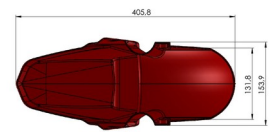
GAMBAR 3. TAMPAK BAWAH
