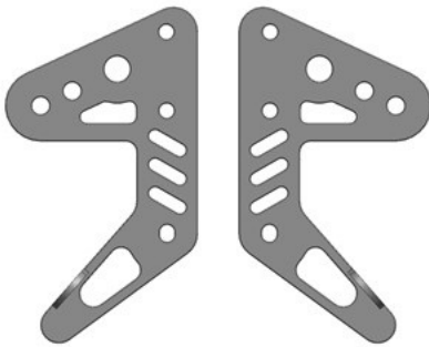
Tampak Belakang
