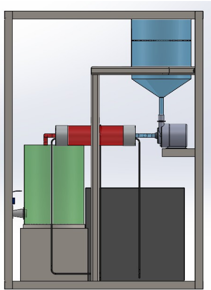
Tampak Belakang
