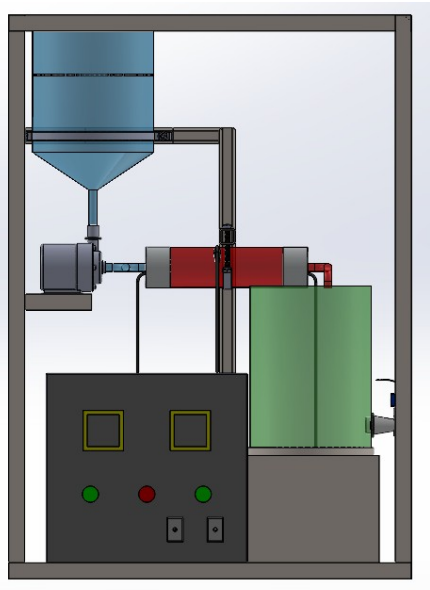
Tampak Depan
