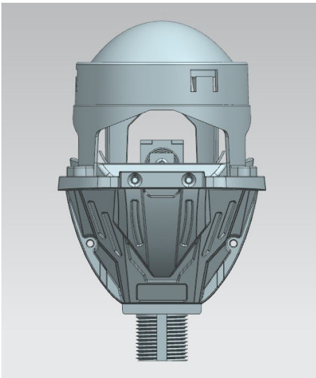
Tampak Atas
