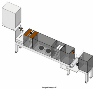
Tampak Perspektif
