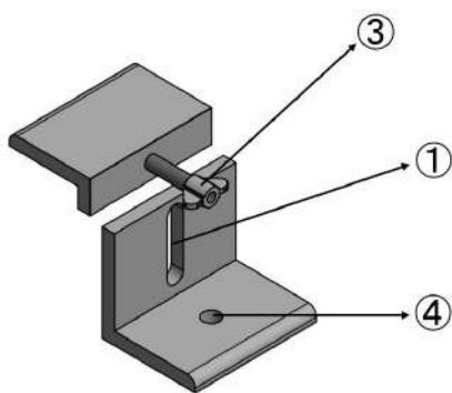
Tampak Perspektif
