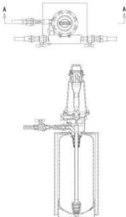
Tampak Atas
