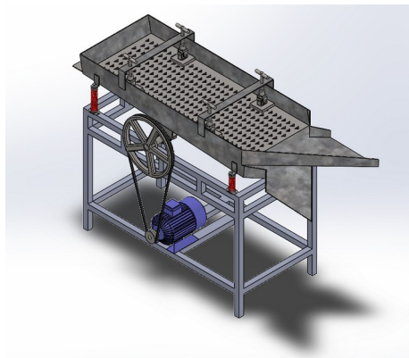
Tampak Perspektif
