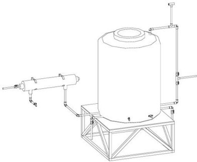
Tampak Perspektif
