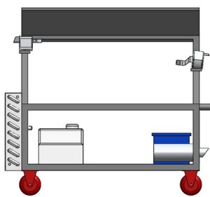
Tampak Depan
