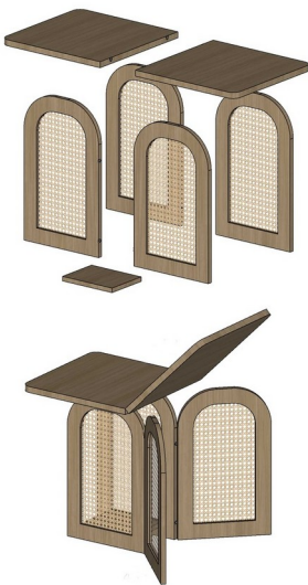
Tampak Perspektif
