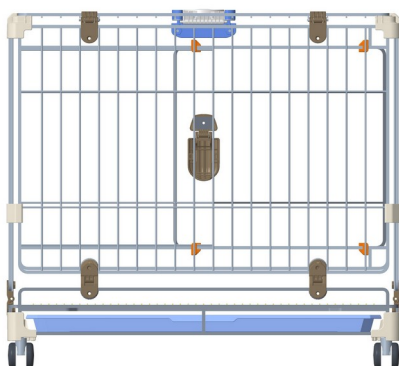
Tampak Belakang
