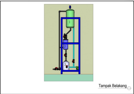
Tampak Belakang
