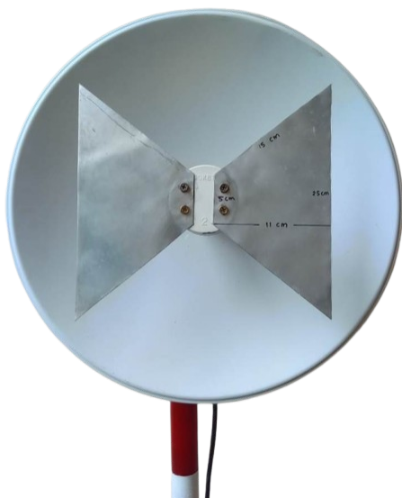
Tampak Perspektif
