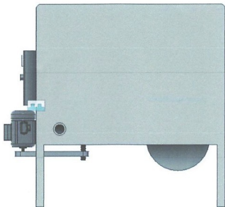
Tampak Belakang
