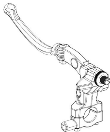
Tampak Perspektif
