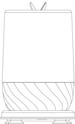
Tampak Depan
